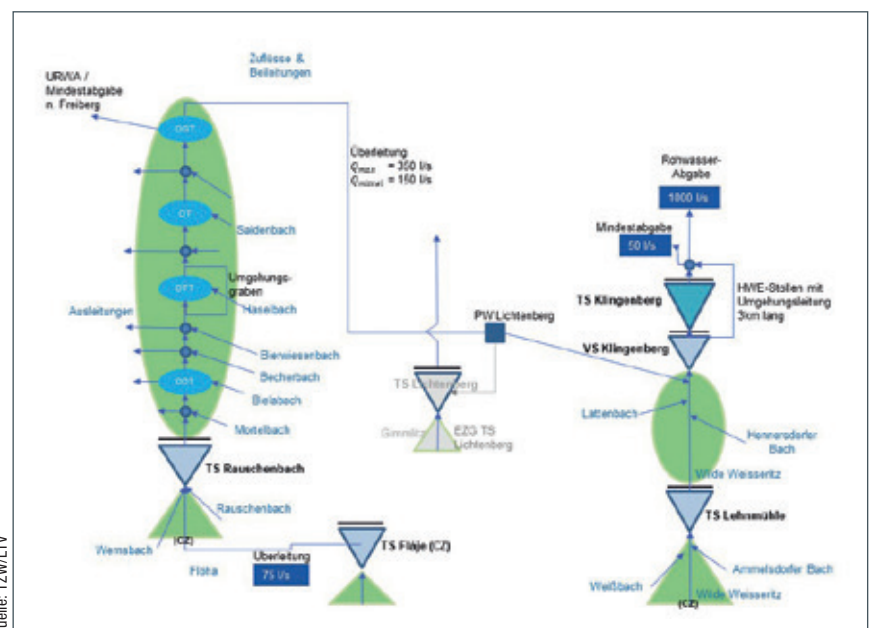
Abb. 1: Schematische Darstellung des Talsperrenverbundes Klingenberg-Lehnmühle-Rauschenbach/ORWA
